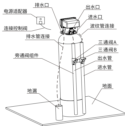
净水器安装示意图
