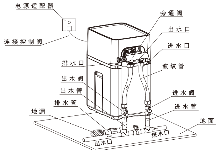
净水器安装示意图
